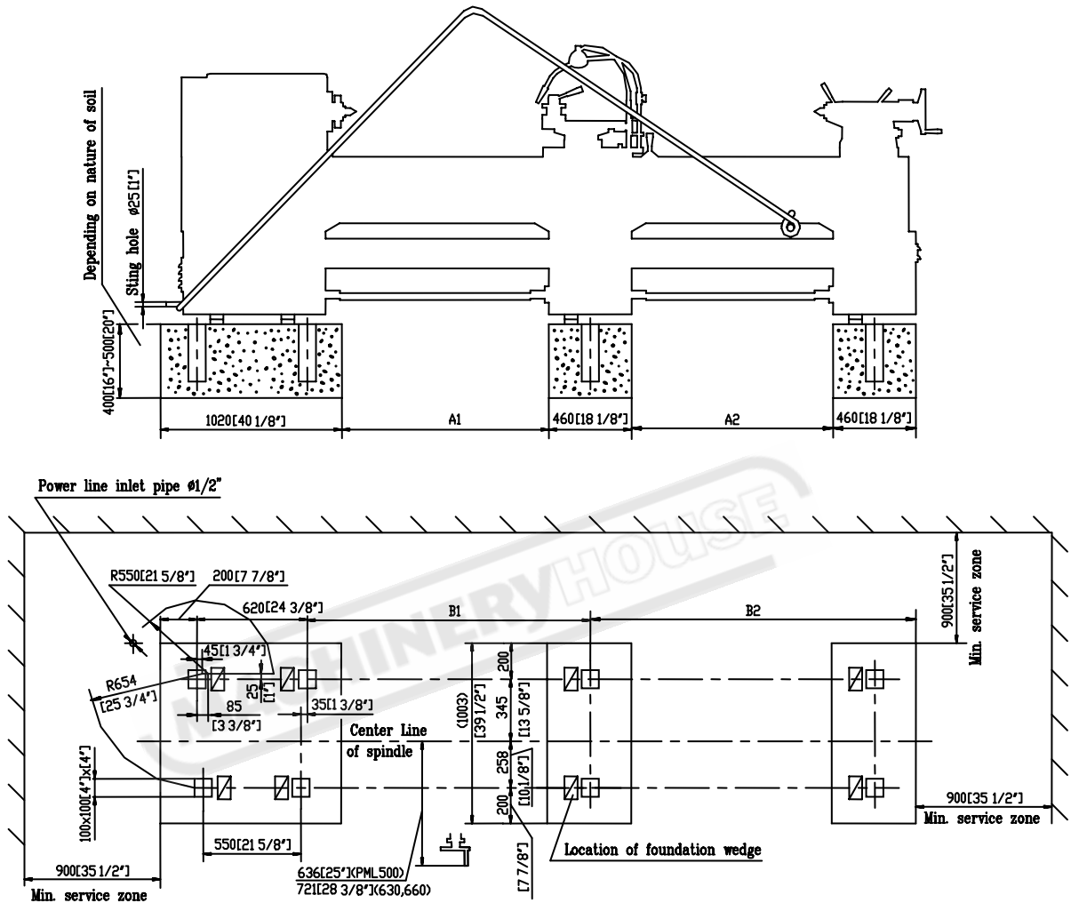
Fig 3-1 2/Lc=2000[80" ]~3000[120" ]
