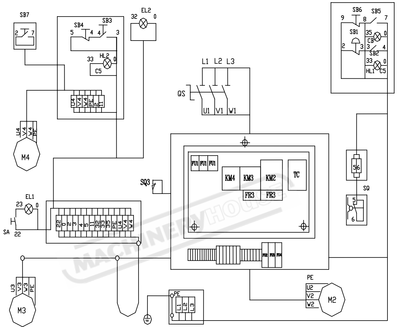
Wiring diagram(图6)
